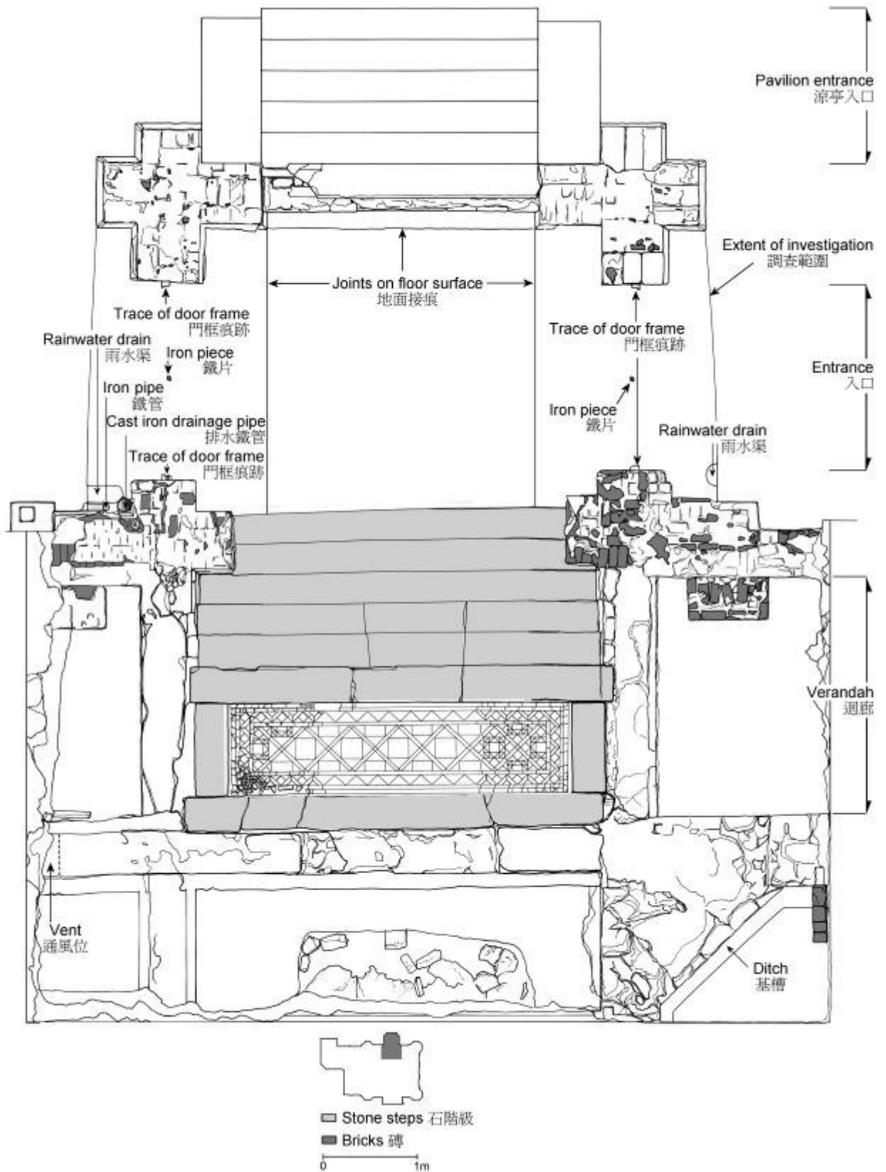
圖 7 入口平面圖 Fig 7 Entrance plan
