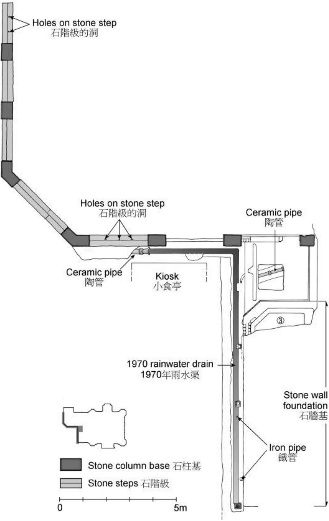
圖 13 探溝 T9 平面圖 Fig 13 Plan of test trench T9
