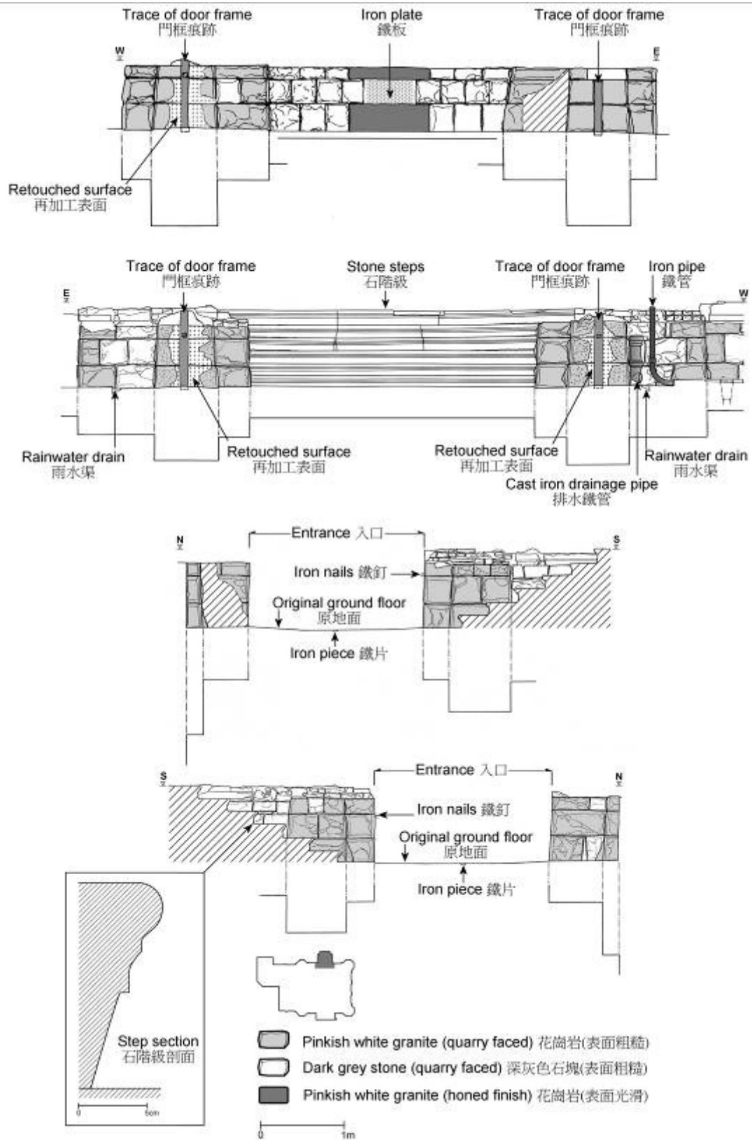
圖 8 入口側視圖
