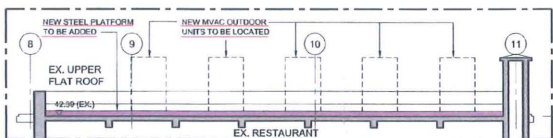
SECTION D-D 1:100
