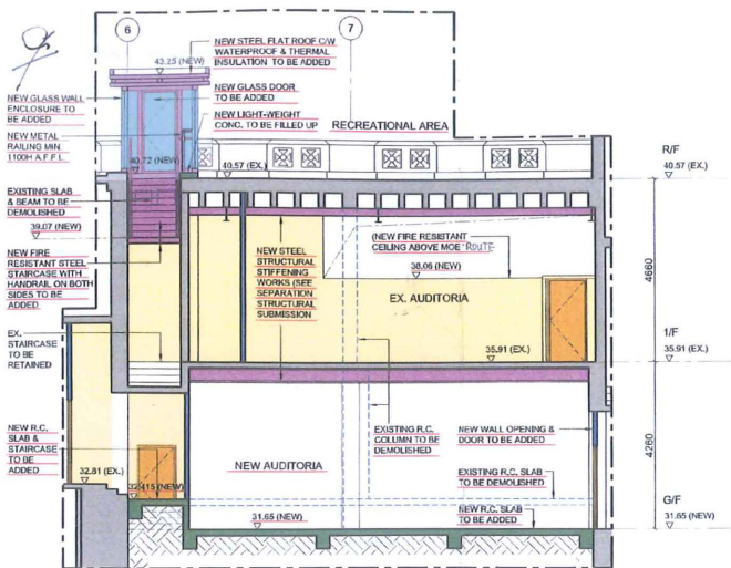
SECTION A-A 1:100
