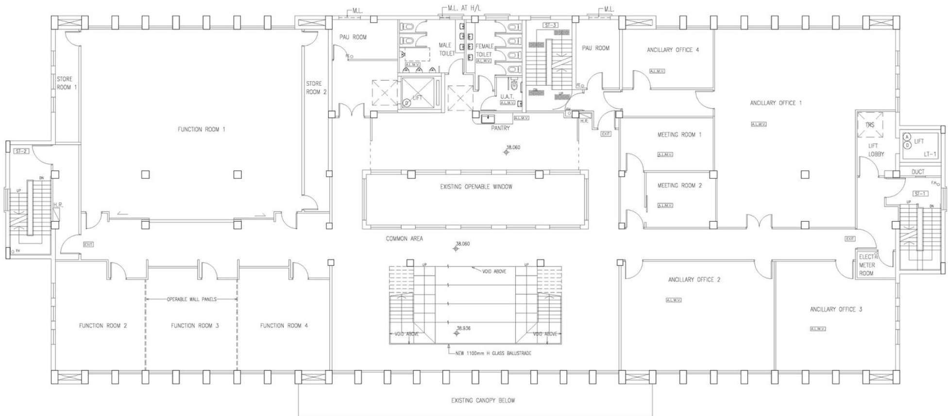
圖 13. 擬議平面圖 —— 四樓
