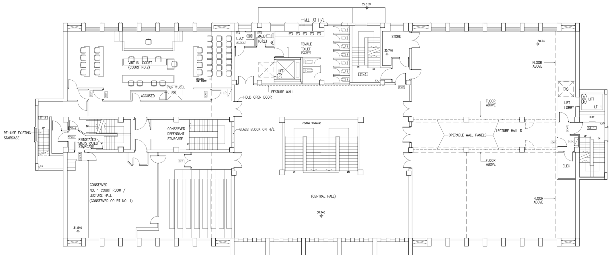
圖 11. 擬議平面圖 —— 二樓
