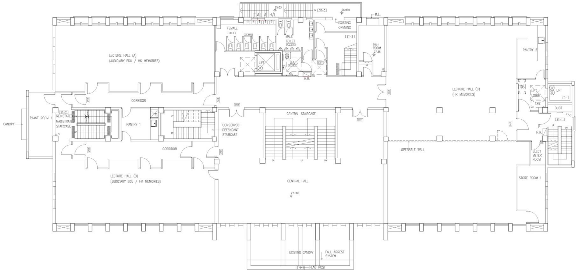
圖 10. 擬議平面圖 —— 一樓
