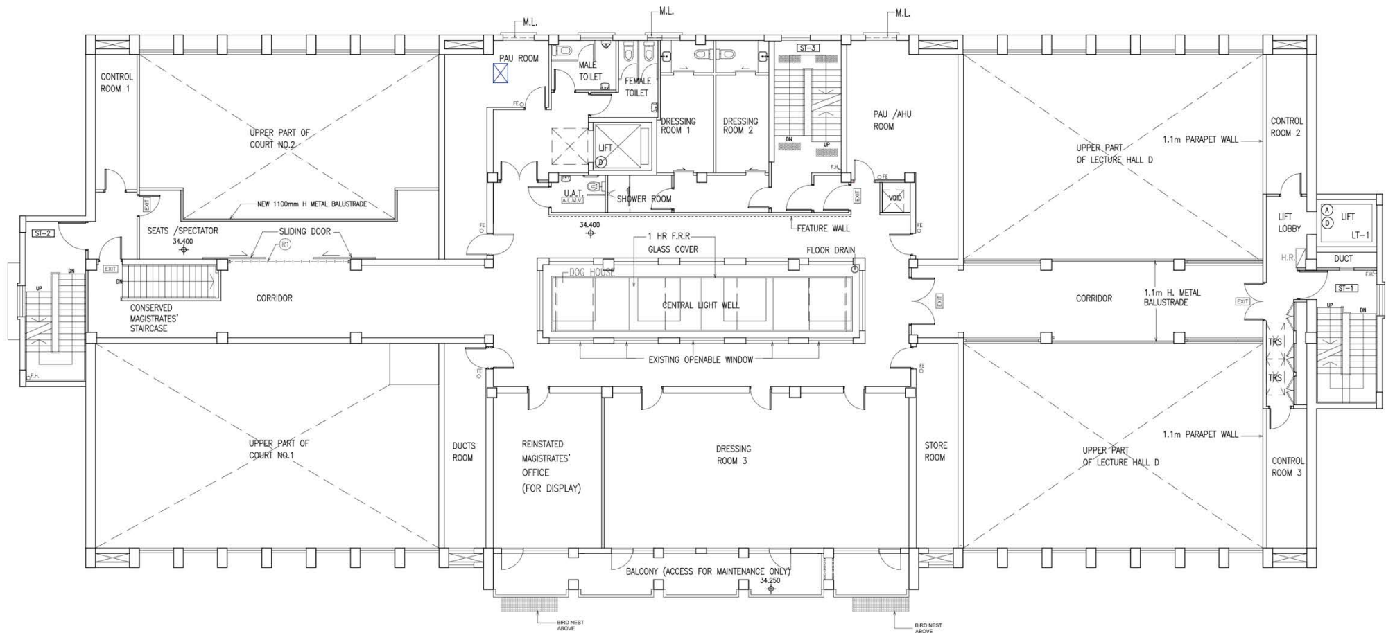
圖 12. 擬議平面圖 —— 三樓
